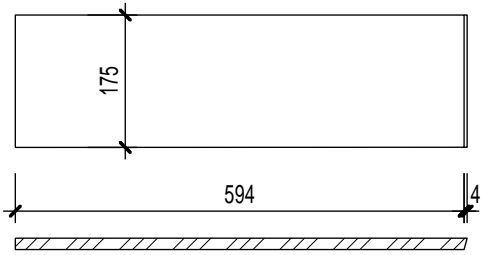
Seitenteil D (Stärke 15 mm) 1 Stk.
