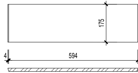
Seitenteil C (Stärke 15 mm) 1 Stk.
