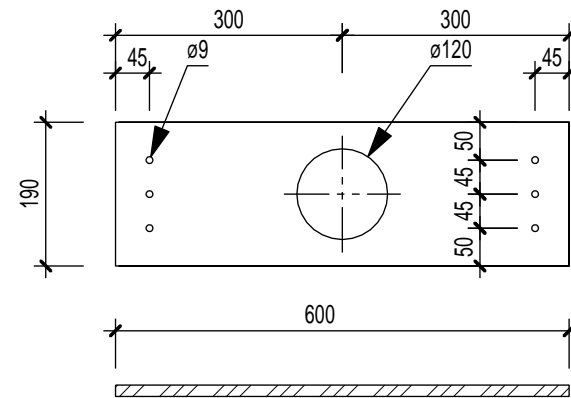
Seitenseite B (Stärke 15 mm) 2 Stk.
